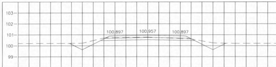
STA. 0+475.000 NGL = 100.780
