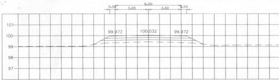
STA. 0+325.000 NGL = 99.430
