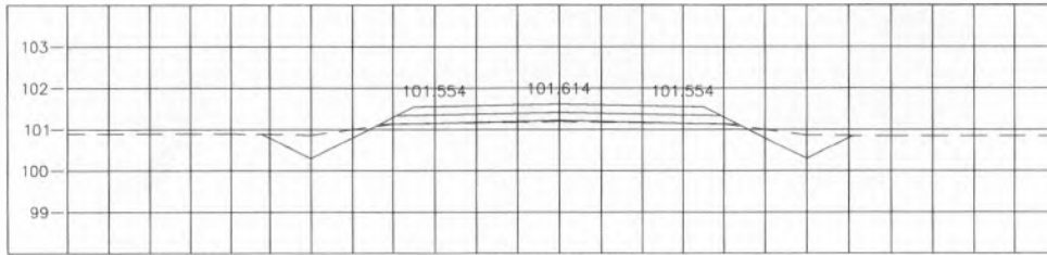
STA. 0+525.000 NGL = 101.195
