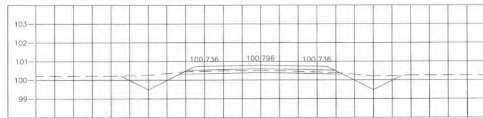
STA. 0+825.000 NGL = 100.515
