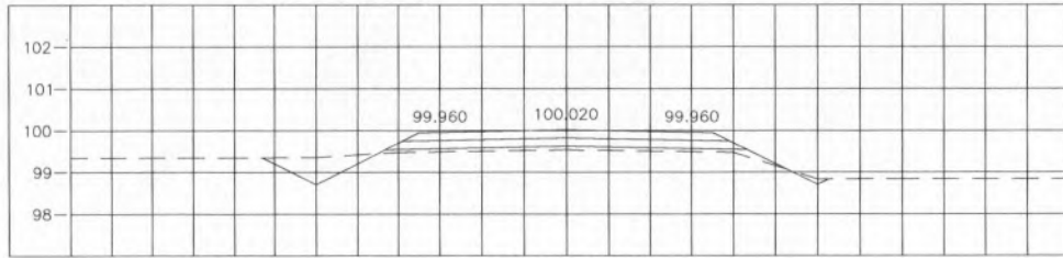
STA. 0+300.000 NGL = 99.530
