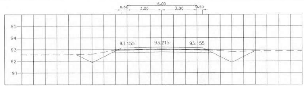
STA. 1+100.000 NGL = 93.065
