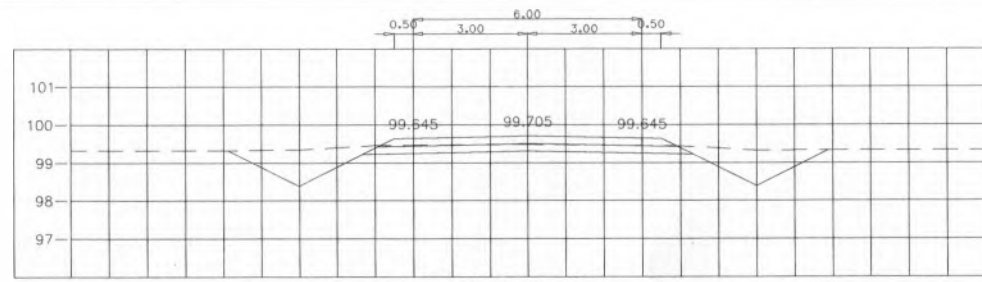
STA. 0+875.000 NGL = 99.485
