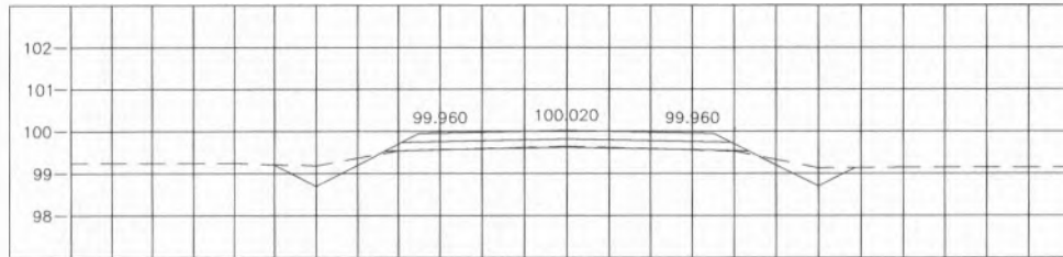
STA. 0+250.000 NGL = 99.640
