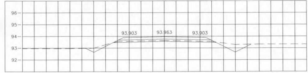
STA. 1+075.000 NGL = 93.645
