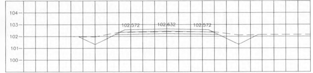
STA. 0+625.000 NGL = 102.395
