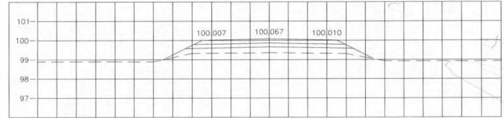
STA. 0+350.000 NGL = 99.360
