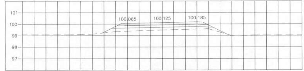
STA. 0+375.000 NGL = 99.490
