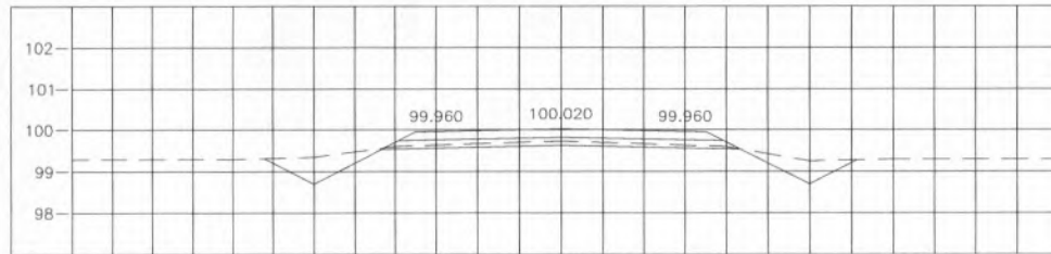
STA. 0+225.000 NGL = 99.730
