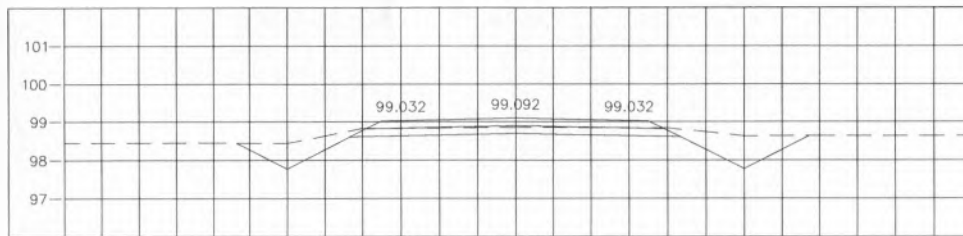
STA. 0+900.000 NGL = 98.855
