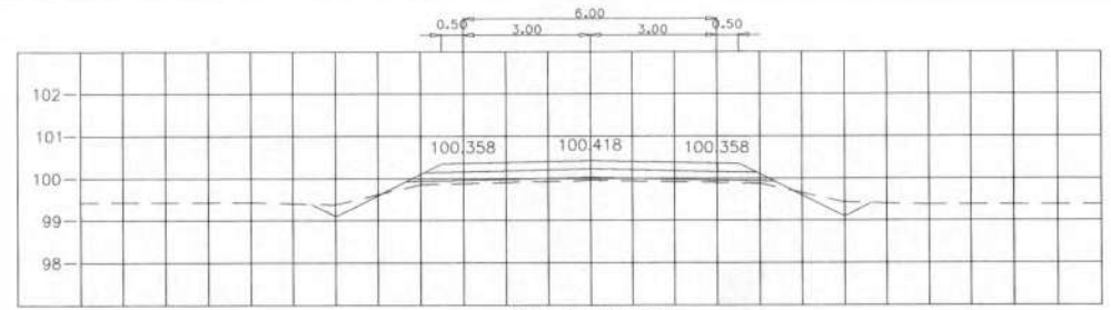
STA. 0+425.000 NGL = 99.950
