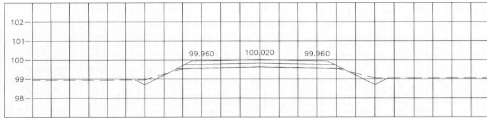
STA. 0+275.000 NGL = 99.630
