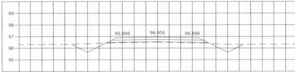
STA. 0+975.000 NGL = 96.505
