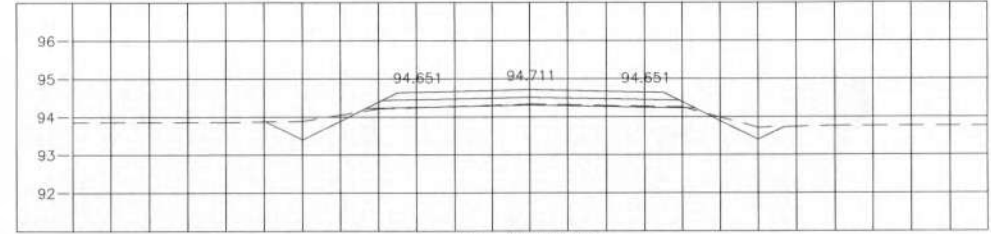
STA. 1+050.000 NGL = 94.335
