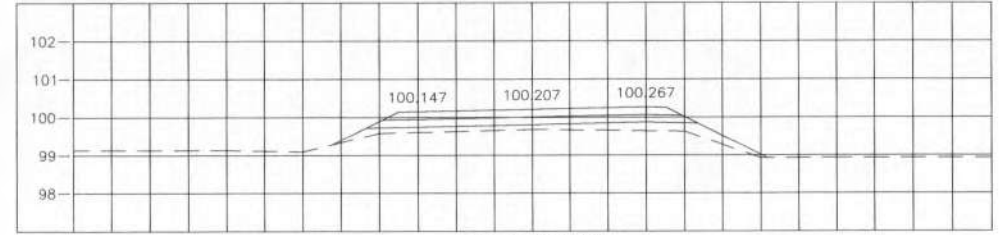
STA. 0+400.000 NGL = 99.680
