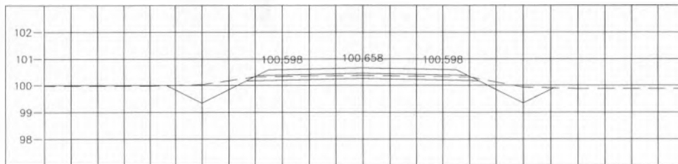
STA. 0+450.000 NGL = 100.380
