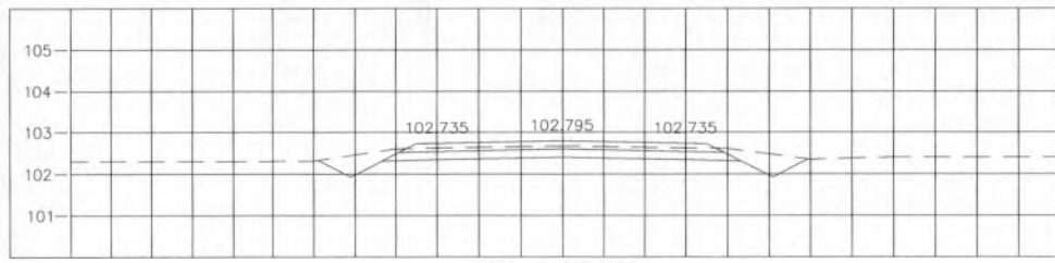
STA. 0+675.000 NGL = 102.670
