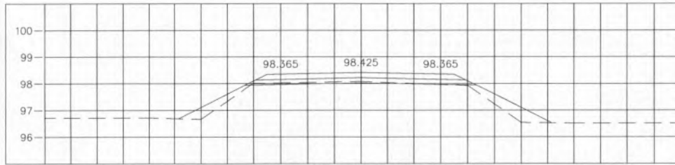
STA. 0+925.000 NGL = 98.085
