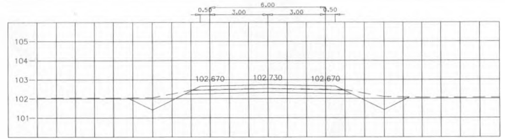
STA. 0+650.000 NGL = 102.535
