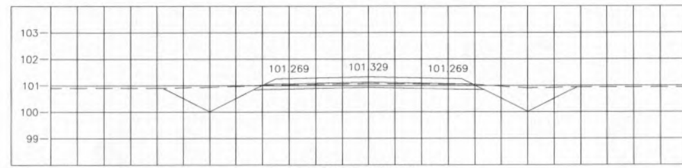
STA. 0+800.000 NGL = 101.075
