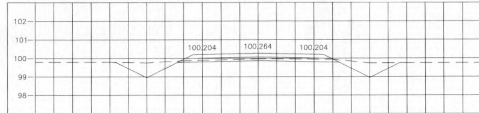
STA. 0+850.000 NGL = 99.965
