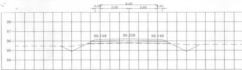
STA. 1+000.000 NGL = 95.775
