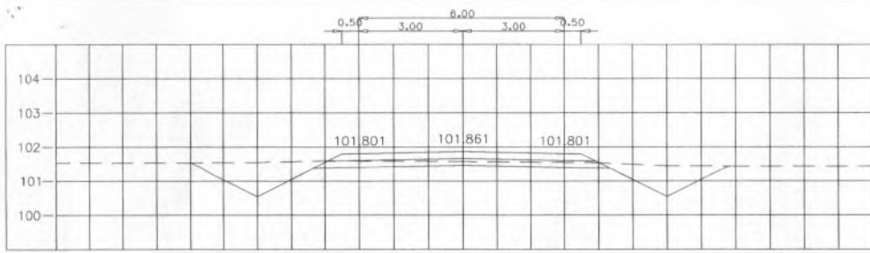
STA. 0+775.000 NGL = 101.575
