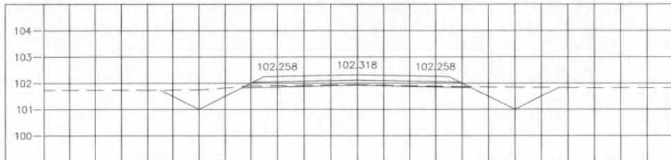
STA. 0+750.000 NGL = 101.935
