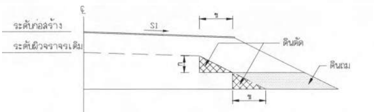
รูปตัดการก่อสร้างลาดคันทางบนถนนเดิม
