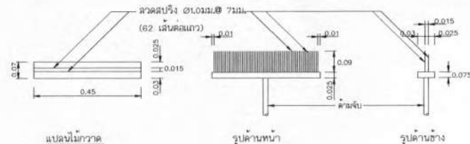
แบบขยายไม่กวดลาดผิวพื้น คสล.
