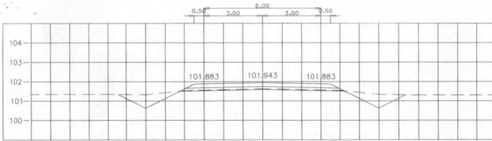
STA. 0+550.000 NGL = 101.625
