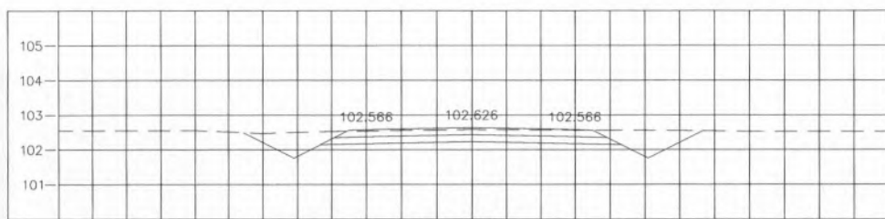
STA. 0+725.000 NGL = 102.575
